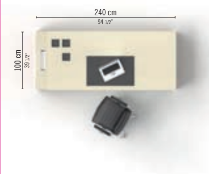
EOS 05 IT Scrivania Direzionale, fin. Bamboo, fianco ad "L" con top access, mobili medi con anta vetro. FR Bureau direction fin. Bamboo, pied "L" avec top access, meubles avec portes en verre. EN Executive desk Bamboo fin., leg with integrated wire management and cabinets with glass doors.
